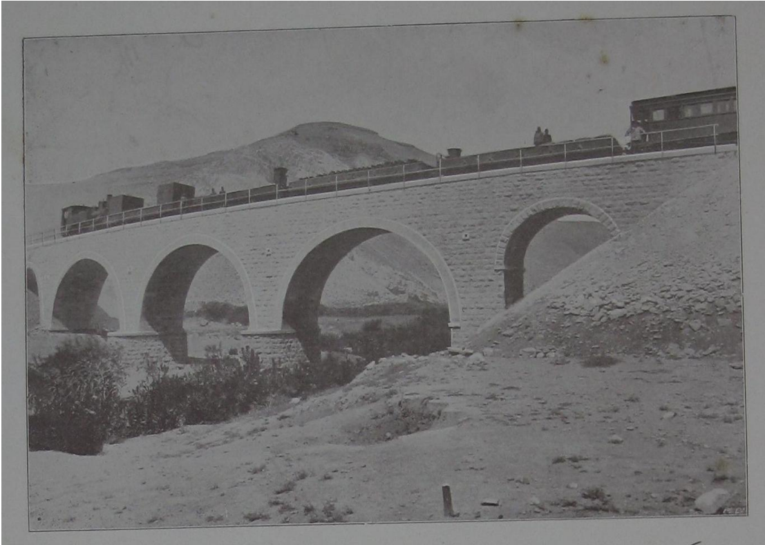
Hayfa hattının 48. Kilomeresinde inşa edilen 48 metre uzunluğunda 6 gözlü köprü 1908(AESLN 235, s.73.)
