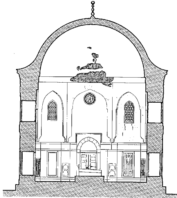
B-B KESİTİ ÖLÇEK 1/50
