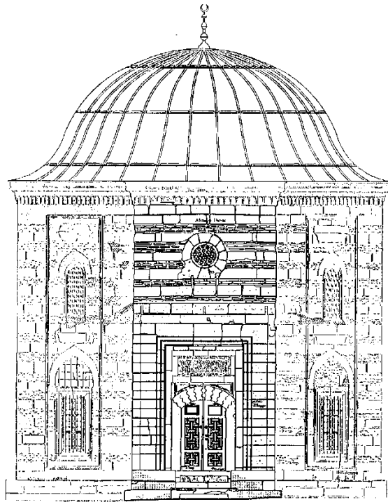
KUZEY CEPHESİ ÖLÇEK: 1/50
