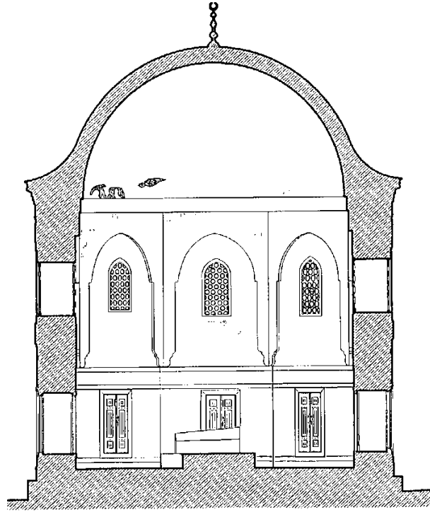
B'-B' KESİTİ ÖLÇEK 1/50
