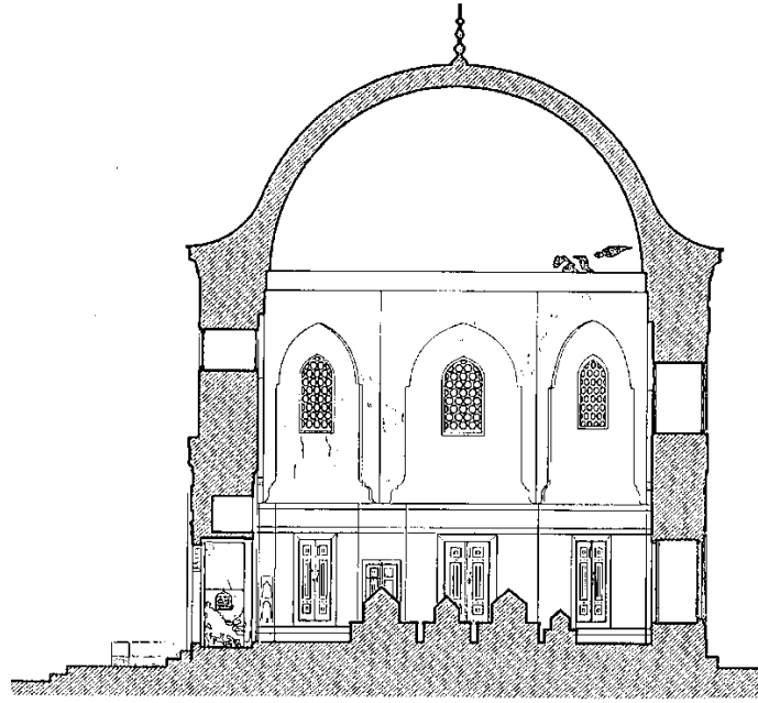
A-A KESİTİ ÖLÇEK 1/50
