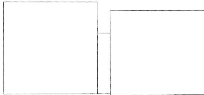
Resim 11: Dromos ve Mezar Odası'nın Boyuna (A-A) kesiti
