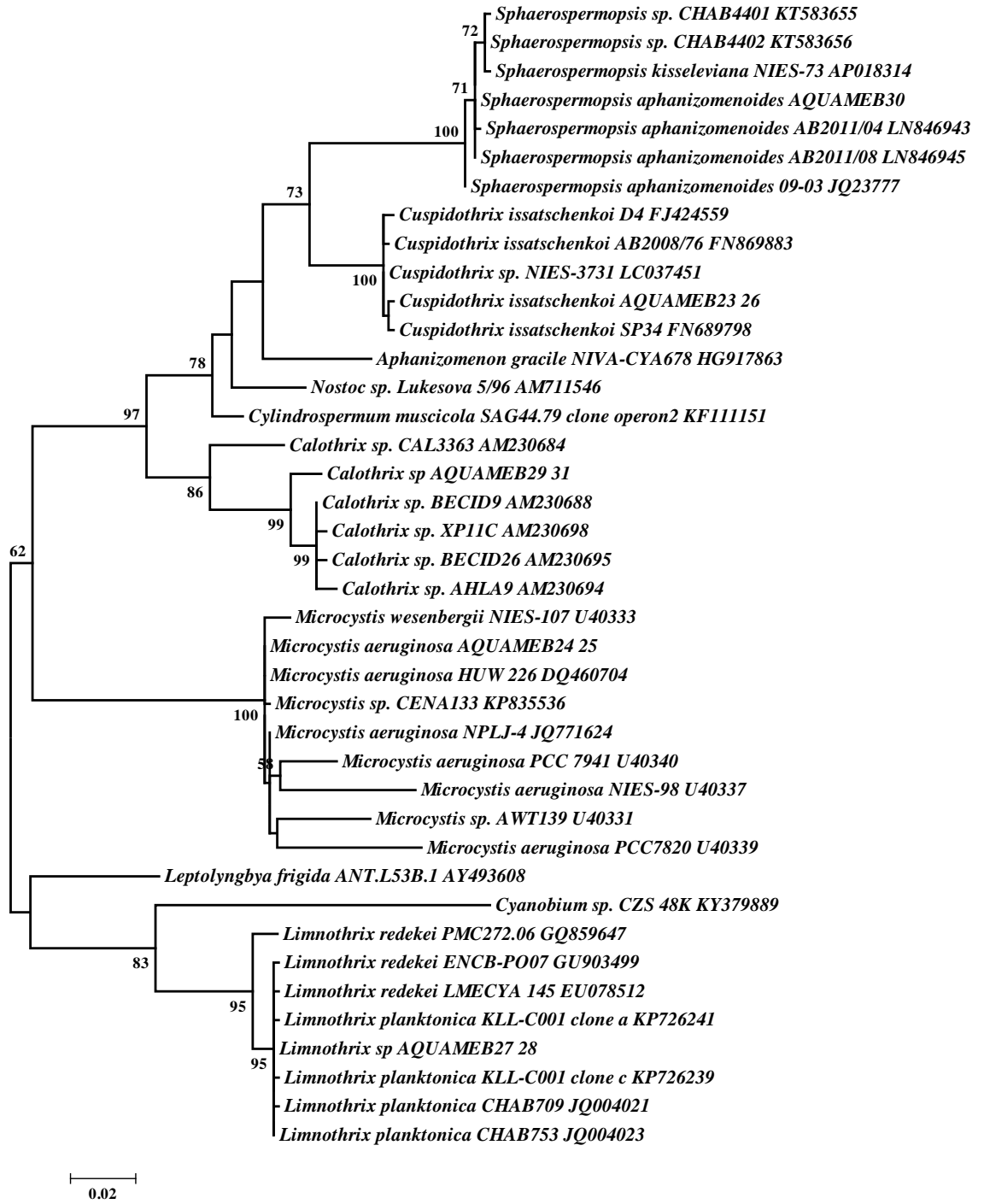
Şekil 4.23. İzole edilen suşların maximum likelihood yöntemi ile oluşturulan 16S rRNA genine dayalı filogenetik ağacı
